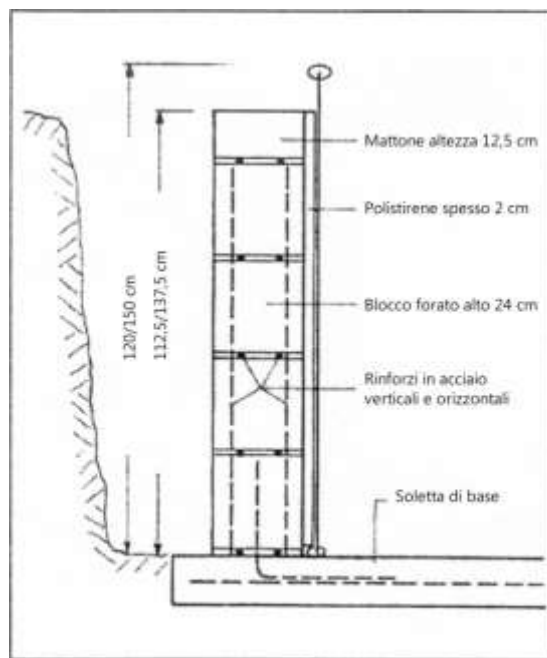
4 blocchi forati + 1 mattone = 112,5 cm per una vasca di 120 cm di altezza 5 blocchi forati + 1 mattone = 137,5 cm per una vasca di 150 cm di altezza
